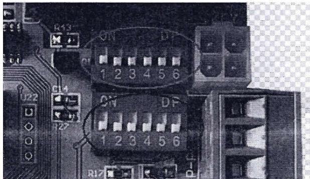
Рисунок 4 – DIP-переключатели
